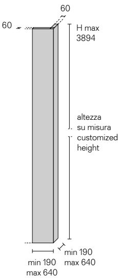
Pannello ad angolo esterno Panel for external corner
